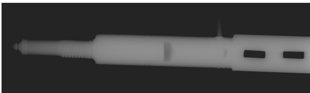
Hřídel kalendářního kola délkově nastavená pravděpodobně v roce 1865 a rentgenové snímky hřídele a vačky mezilehlého kola bicího stroje
