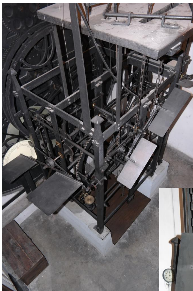
Stroj orloje před restaurováním
