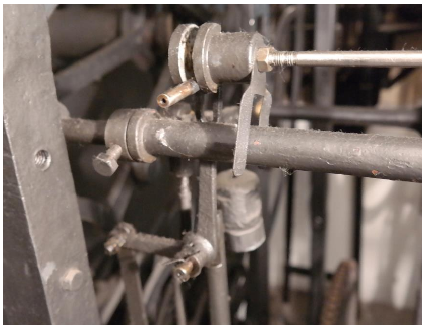
Detail systému regulujícího samostatné vypouštění bicího stroje a společné vypouštění stroje bicího i apoštolského
