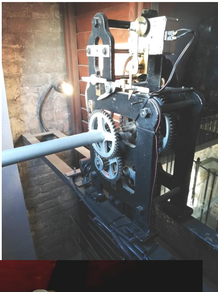
Zrestaurovaný hodinový stroj a podružný stroj u ciferníku
